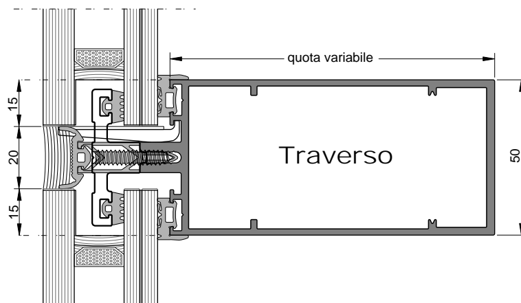
Facciata continua RG (ritegno vetro strutturale)
